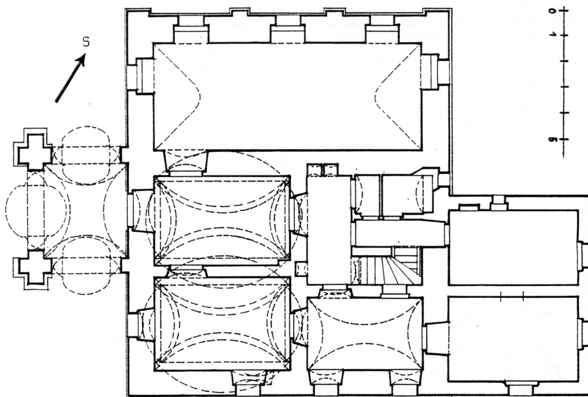
Obr. 2: Kojšice. Půdorys přízemí zámku
