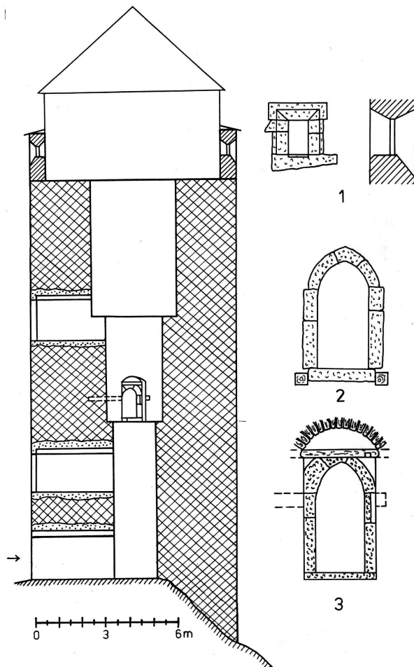
Obr. 2 – Hasištejn (okr. Chomutov). Řez bergfritem (označení stáří zdiv viz obr. 1) a detaily: 1 – nákras ostění renesanční střílny při pohledu z interiéru věže a řez střílnou, 2 – vstupní portálek do věže při pohledu z exteriéru, 3 – vstupní portálek do věže při pohledu z interiéru. Rozlišení stáří zdiv viz popiska obr. 1.
