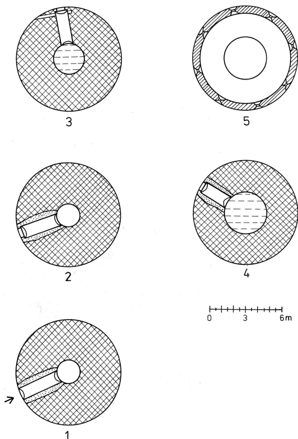
Obr. 1: Hasištejn (okr. Chomutov). Půdorysy jednotlivých podlaží bergfritu. Křížkované zdivo z počátku 14. století, šrafované zdivo z přelomu 15. a 16. století, tečkované zdivo z let 1891 – 1892.
