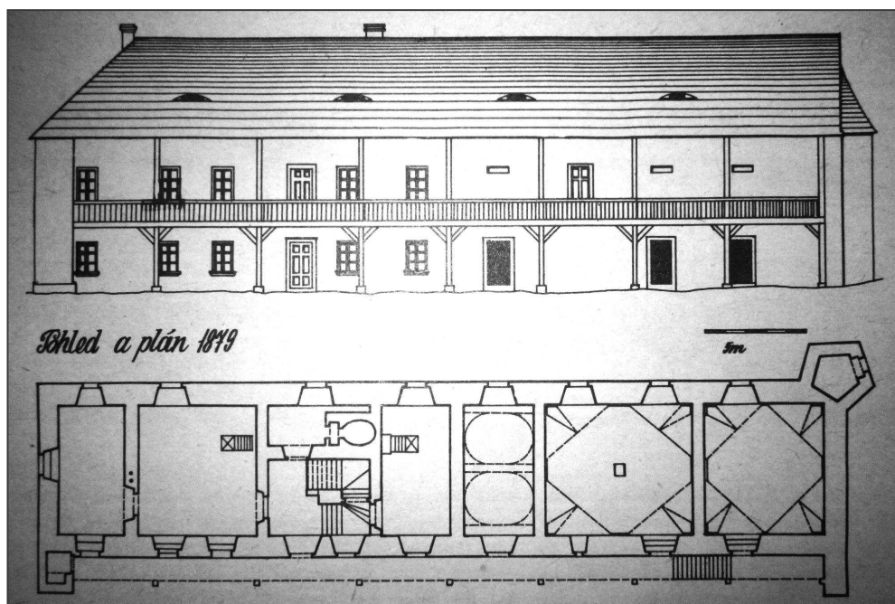
Plán zámku Gutštejn-Daňkov před úpravou z r. 1879 (SOA Plzeň, Vs Bezručice, plán č. M 35; kresba Z. Procházka 1988).
