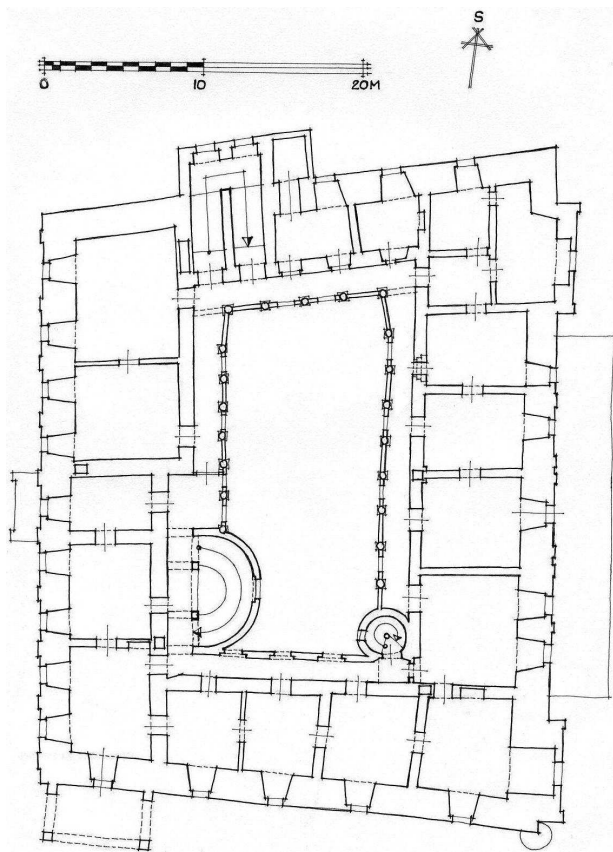
Obr. 4. Půdorys prvního patra zámku dosud vymezuje středověká obvodová zeď, čitelné jsou i gotické a pozdně gotické palácové budovy přiložené k vnitřním lícům hradby v severní části nádvoří.
