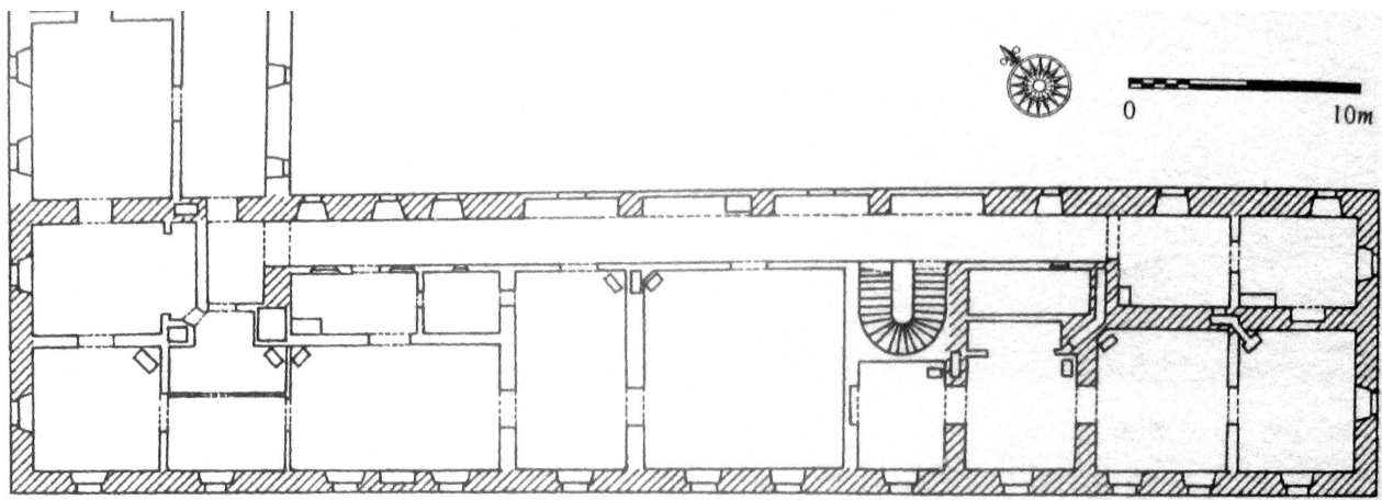
Přízemí jižního (jihozápadního) křídla zámku na plánu z doby kolem r. 1900. Šrafovaně předpokládané renesanční zdivo (kresba J. Úlovec, Kolektiv: Encyklopedie českých tvrzí II. Praha 2000, s. 306).
