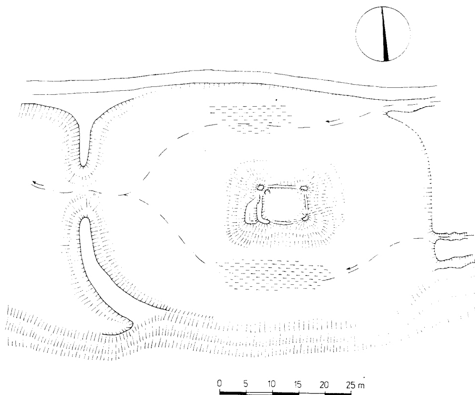
Obr. 1: Půdorys tvrziště u Turyňské hájovny (zaměřili autoři a M. Ebel, stav únor 1985).
