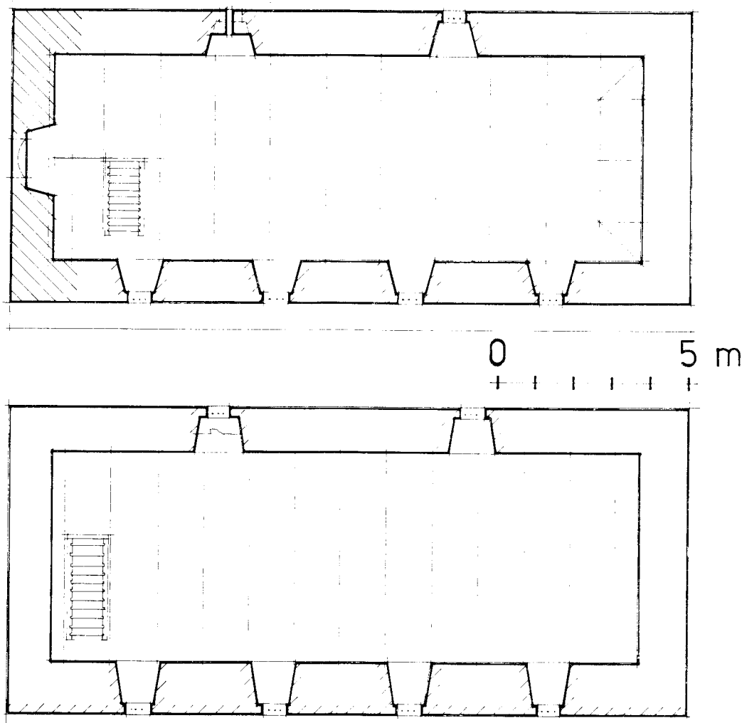
Obr. 3: Řesanice. Palác tvrze - 3. a 2. nadzemní podlaží objektu.
