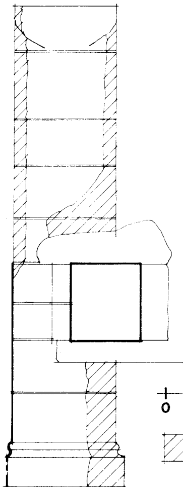
Obr. 3: Kost - situace po odstranění omítek z původního nároží bieberštejnského paláce.
