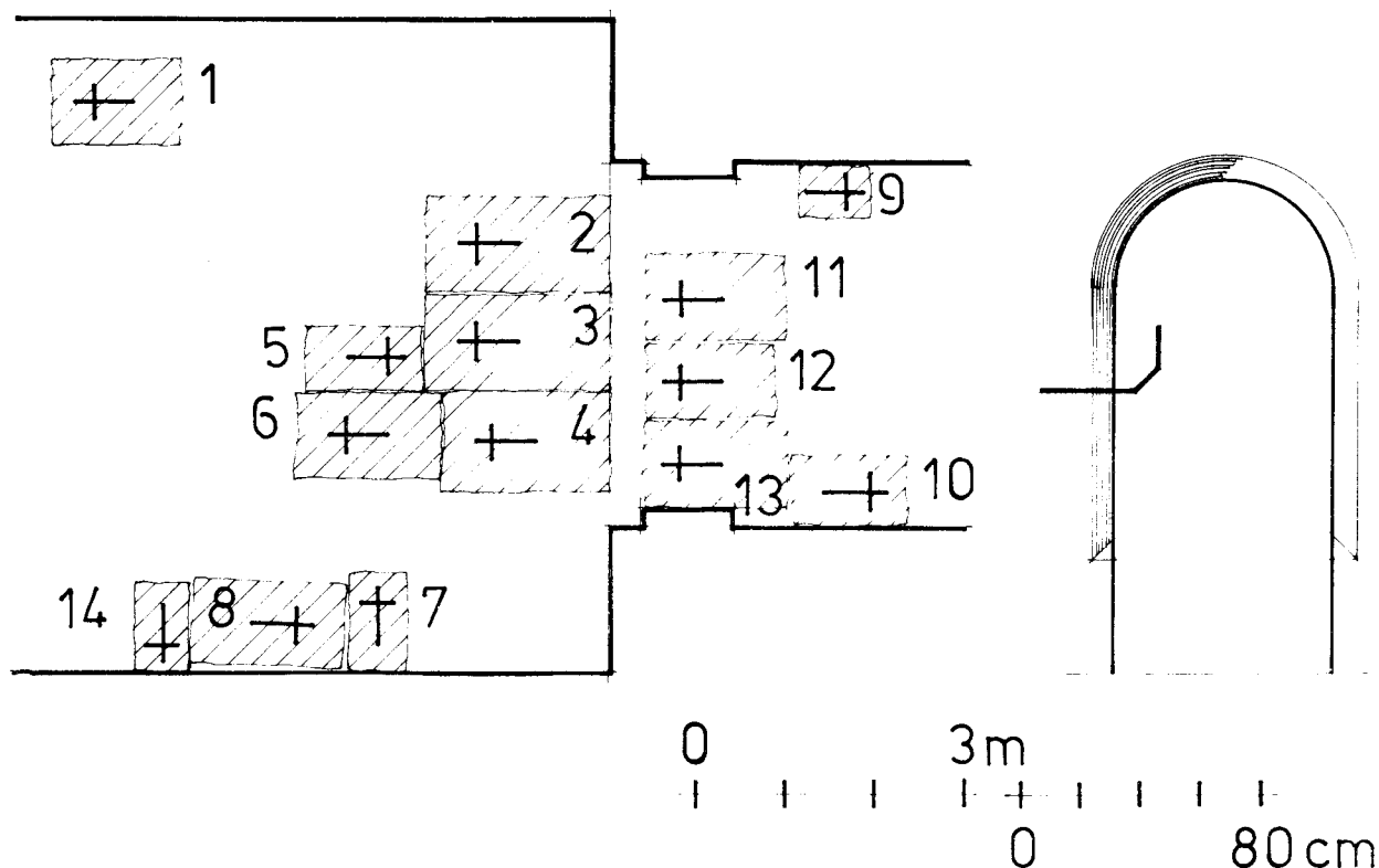
Obr. 7: Řesanice, kostel Věch svatých. Situace náhrobků a branka v ohradní zdi.
